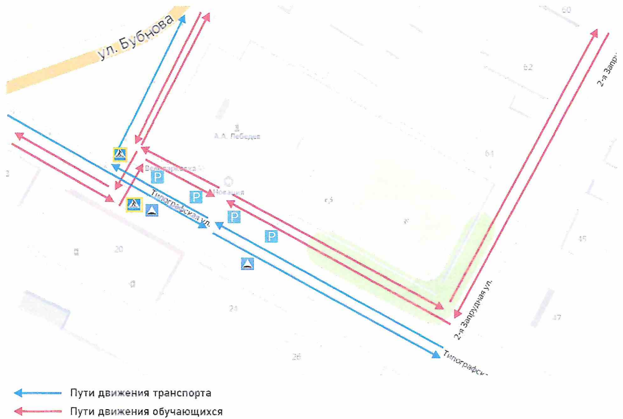
2.2 Схема организации дорожного движения в непосредственной близости от ОУ с размещением соответствующих технических средств, маршруты движения обучающихся и расположение парковочных мест
